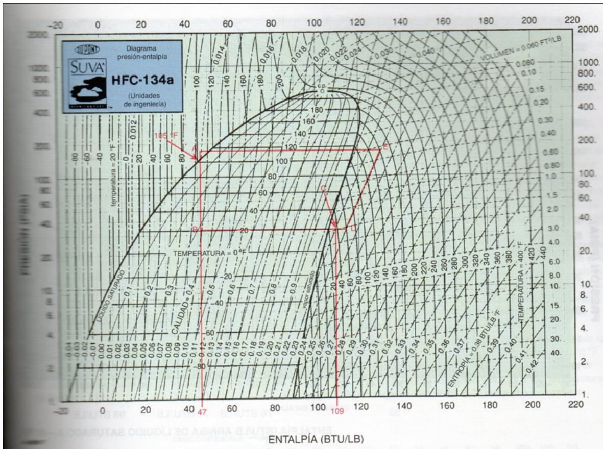
Diagrama de Presión-Entalpía del refrigerante HFC-134a.
